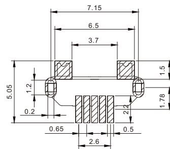
安装图 Instructions
