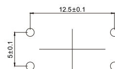
安装图 instructions
