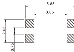
安装图 instructions
