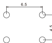
安装图 instructions
