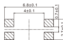
安装图 instructions
