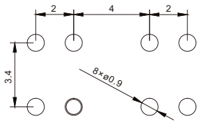
安装图 instructions
