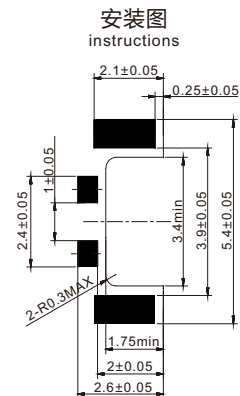
安装图 instructions
