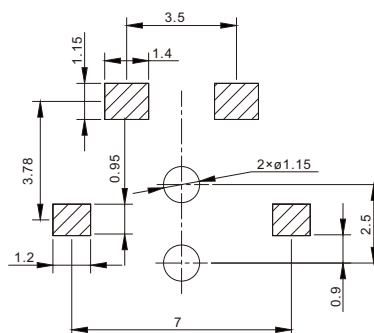
安装图 instructions
